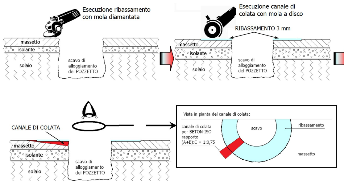
Fig. 3: esecuzione del ribassamento e del canale di colata per BETON ISO
