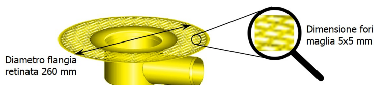
Fig. 1: immagine del POZZETTO SCARICO LATERALE SIFONATO
